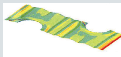
Коеф. тепловіддачі. Вт/м²·К
